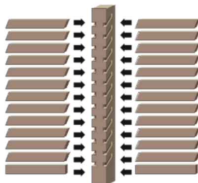
# Poteau intermédiaire entaillé 2 faces
